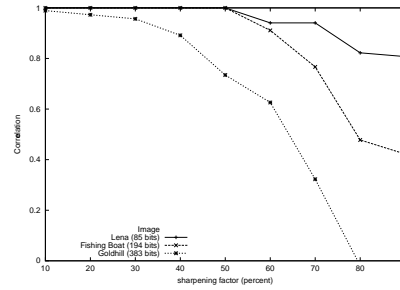
(d) sharpen
